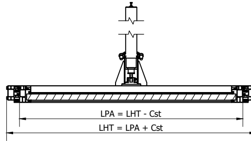
A-A ( 1:10 )
